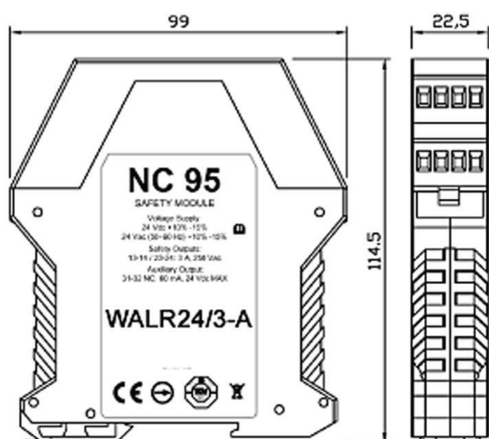
NC95 Dimensioni
